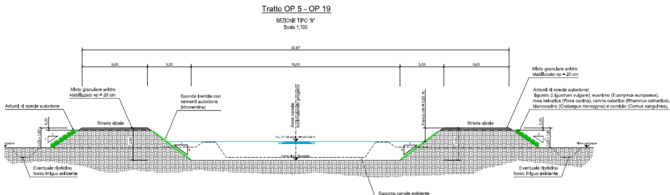
Figura 4 – Esempio di sezione tipo del canale scolmatore in progetto
